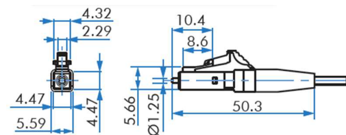
LC „short boot“ Steckverbinder
