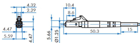
LC Ø2.0mm Steckverbinder
