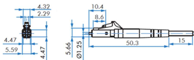
LC Steckverbinder
