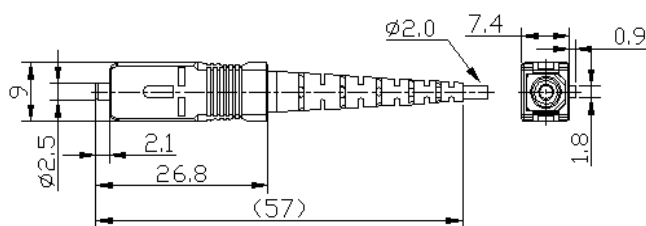
SC Steckverbinder
