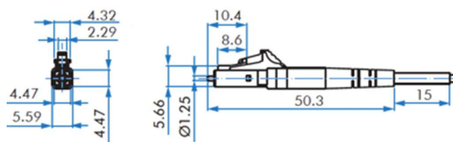
LC Steckverbinder
