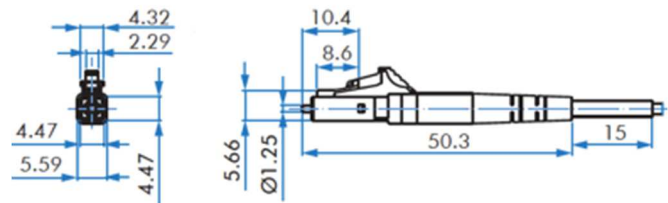
LC Steckverbinder
