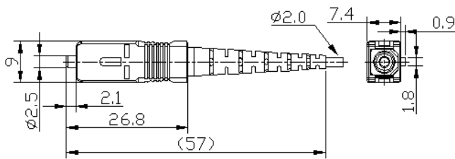
SC Steckverbinder
